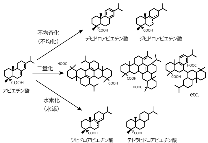
図4 安定化反応
