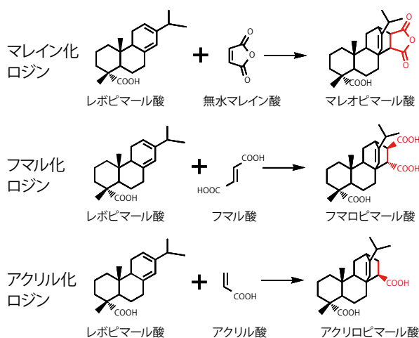
図2 ディールスアルダー付加反応
